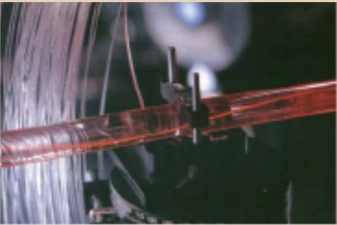
GI 型 POF の原理を示すレーザービームの蛇行
